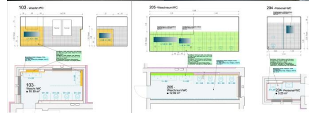
Sanitär-/Wickelbereiche, Fliesenpläne
