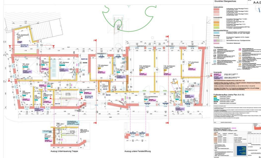
Lageplan, Grundriss Erd- und Obergeschoss
