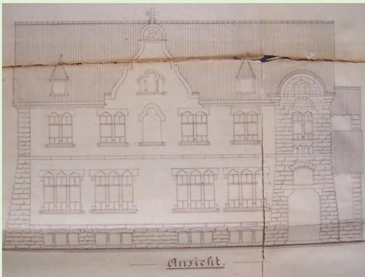
Neubau Kinderbewahranstalt 1904, Auszug Bauakte des Fürstlich Schwarzburgischen Landratsamtes Frankenhausen
